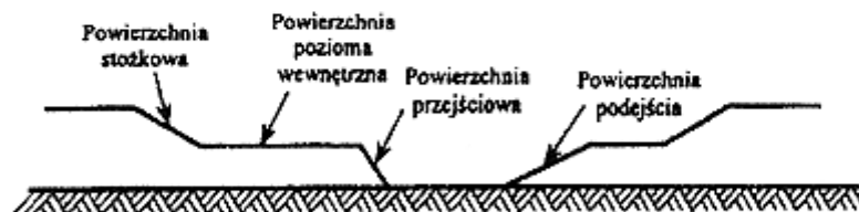
PRZEKRÓJ A-A
