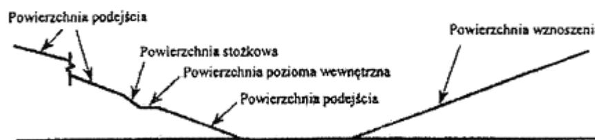
PRZEKRÓJ A-A
